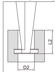
被测尺寸(使用下爪)
